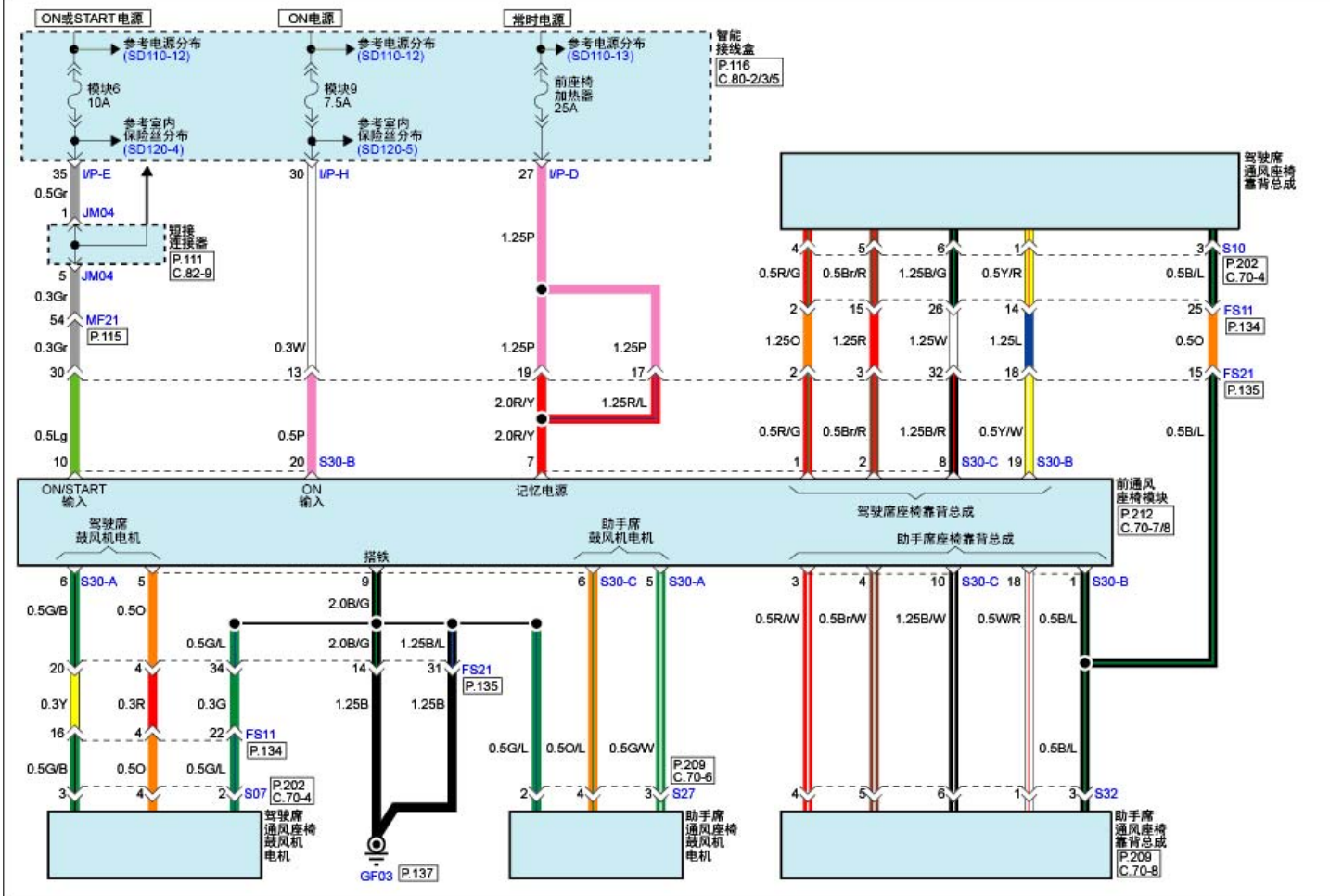
通风座椅控制系统(1)
